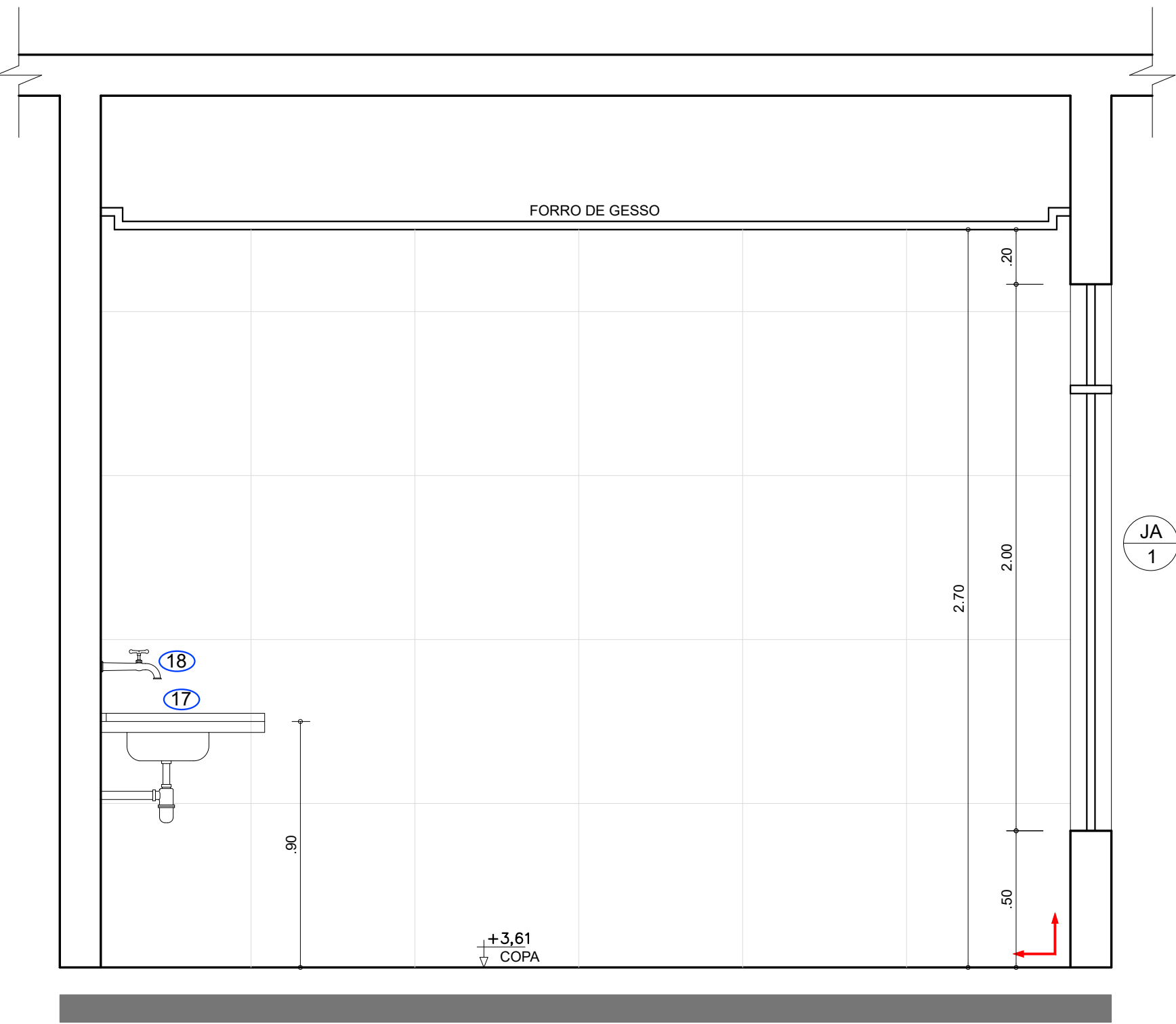
VISTA 1 — COPA PAV. TÉRREO ESC.: 1:25
