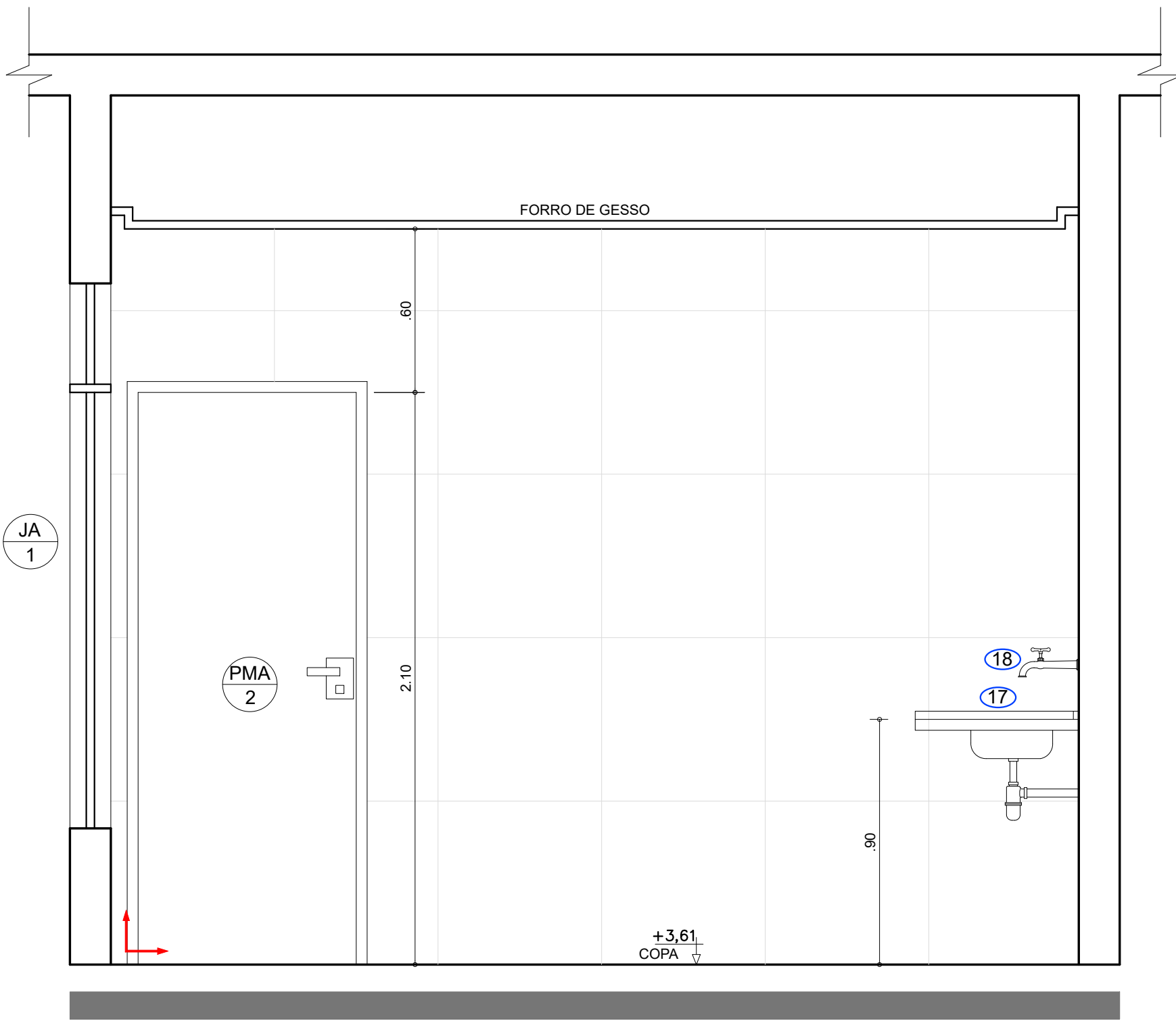
VISTA 2 — COPA PAV. TÉRREO ESC.: 1:25
