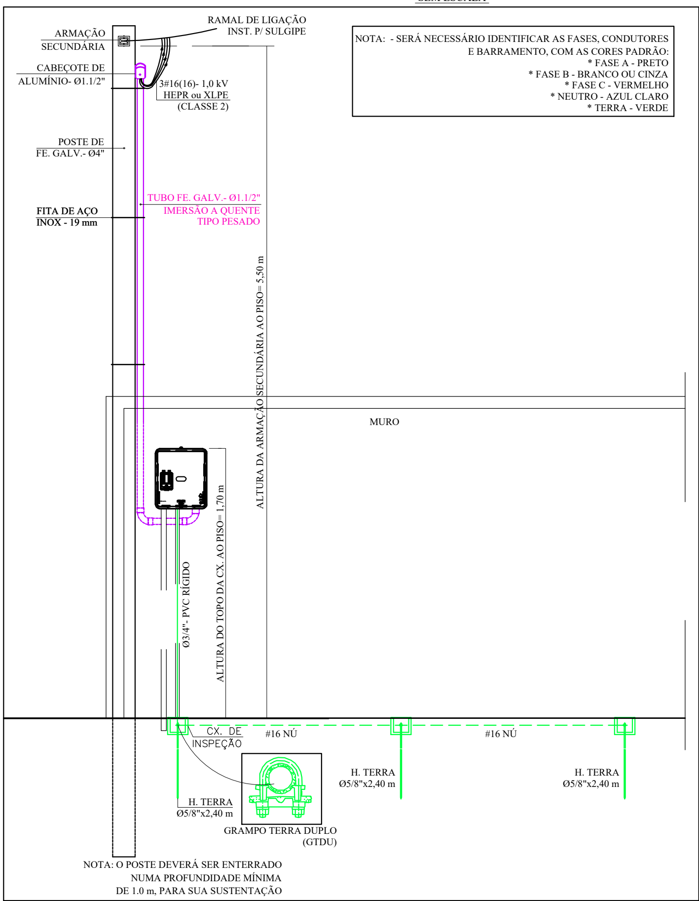
DETALHE DE ENTRADA / MEDIÇÃO SEM ESCALA
