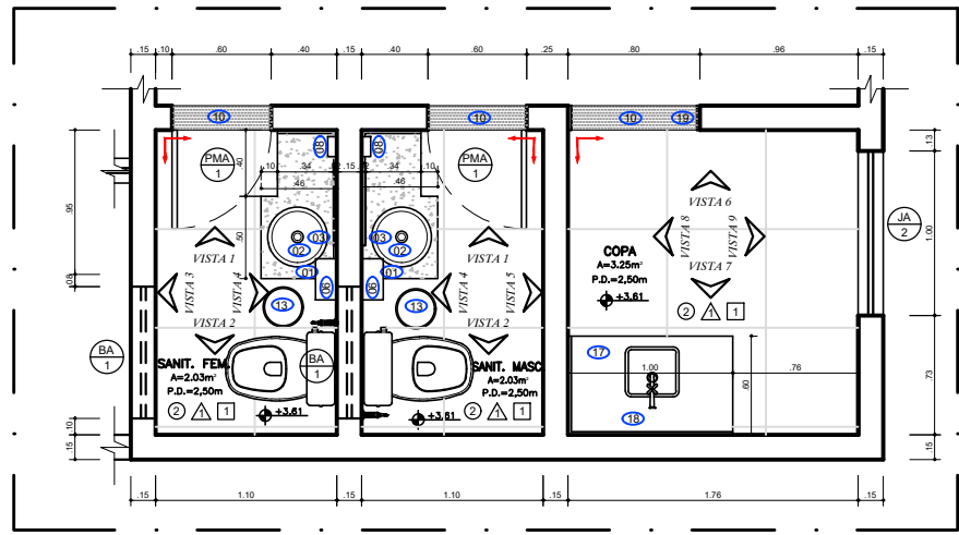
PLANTA BAIXA - SANITÁRIOS DO PAV. SUPERIOR
