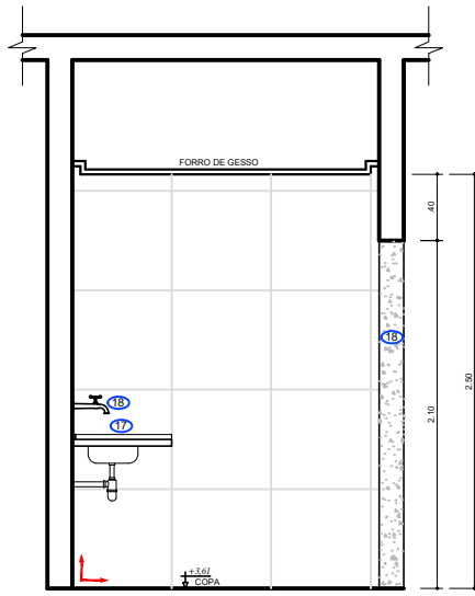
VISTA 6 - SANITÁRIOS PAV. SUPERIOR
