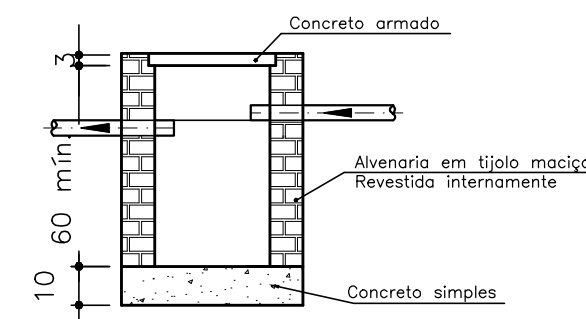
CORTE 2-2
