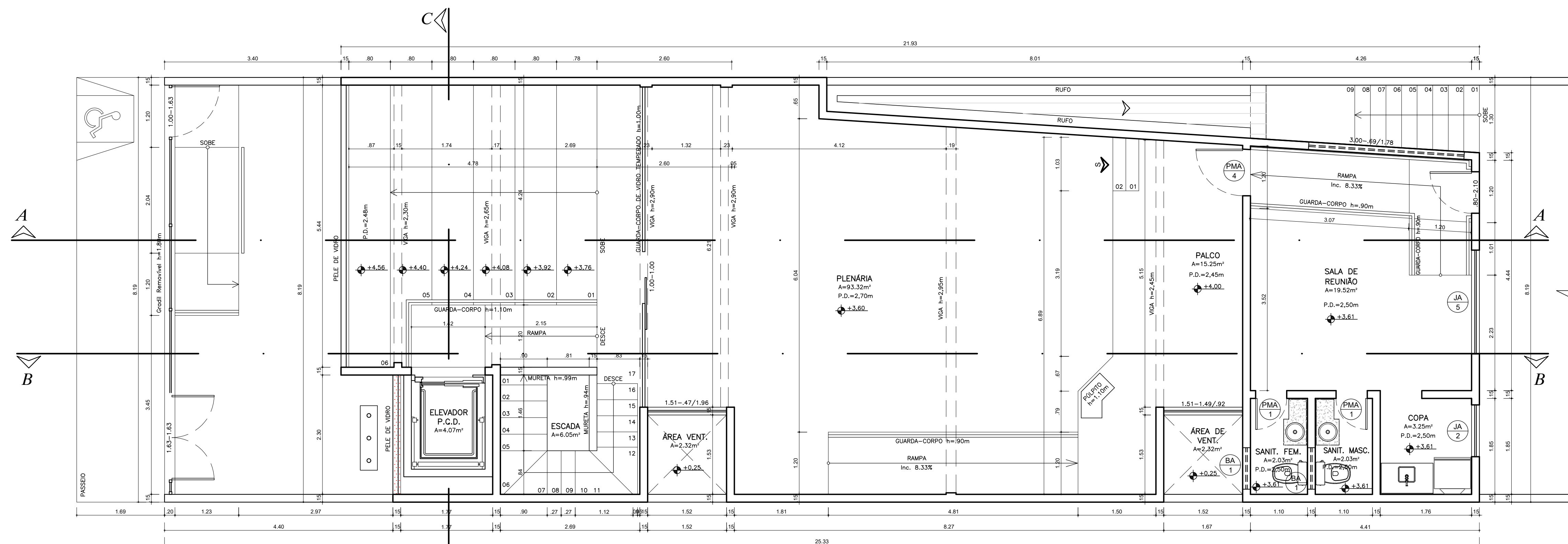
PLANTA BAIXA-PAV. SUPERIOR
