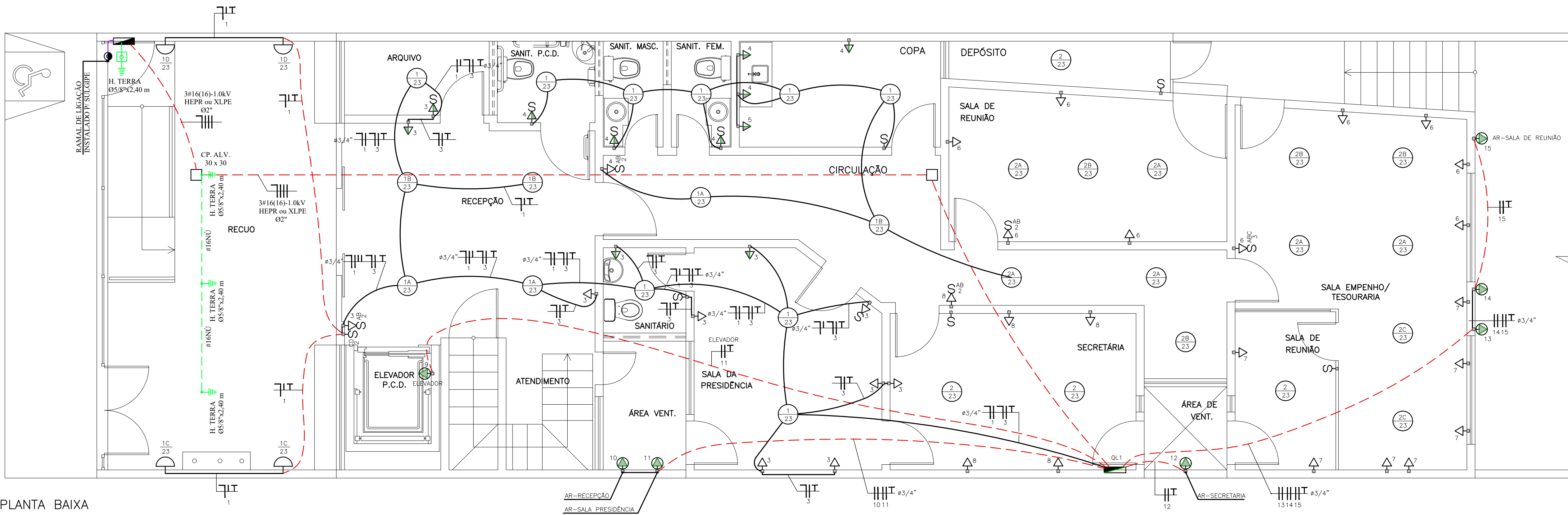
PLANTA BAIXA PAV. TÉRREO ESCALA 1/50
