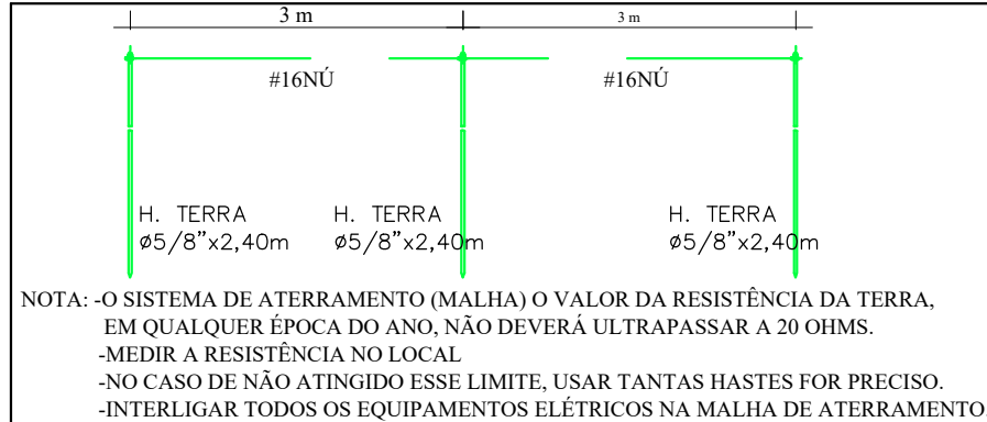
DET. DA M. DE ATERRAMENTO (USO INTERNO) SEM ESCALA
