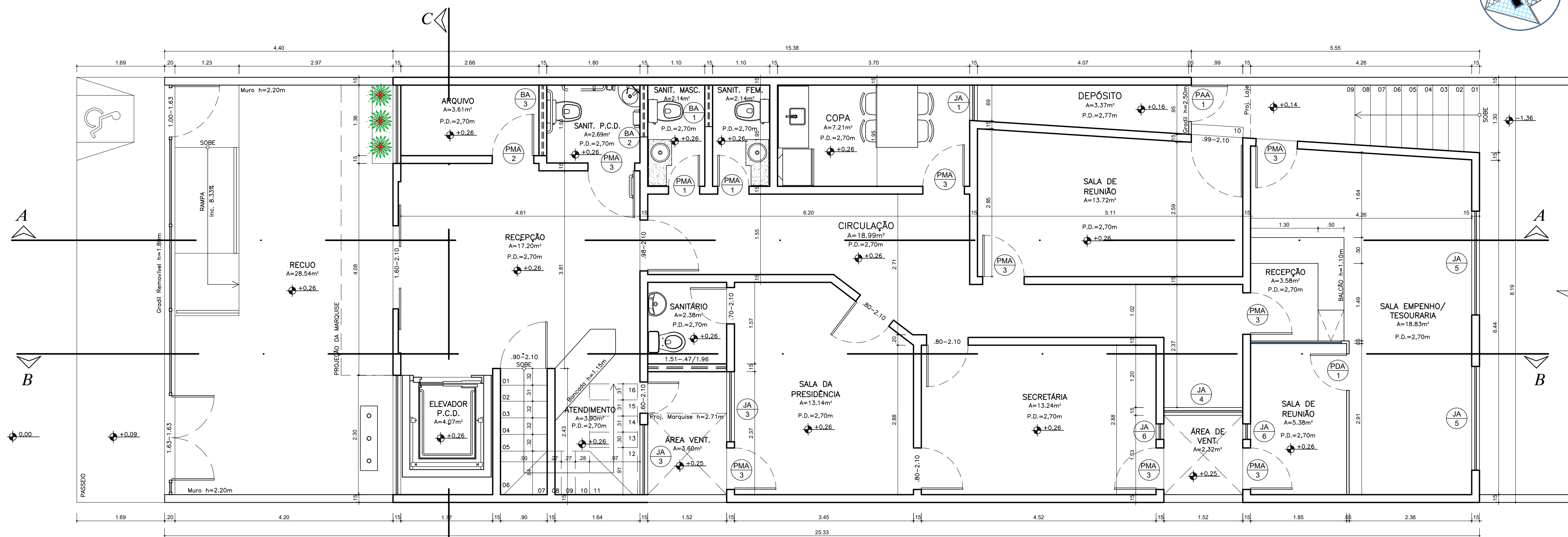
PLANTA BAIXA-PAV. TÉRREO
