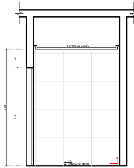
VISTA 5 - SANITÁRIOS PAV. SUPERIOR
