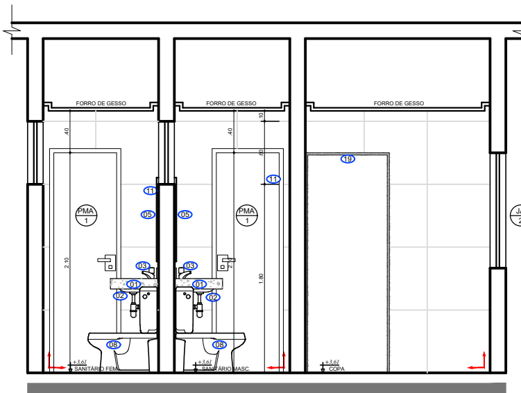
VISTA 1 - SANITÁRIOS PAV. SUPERIOR
