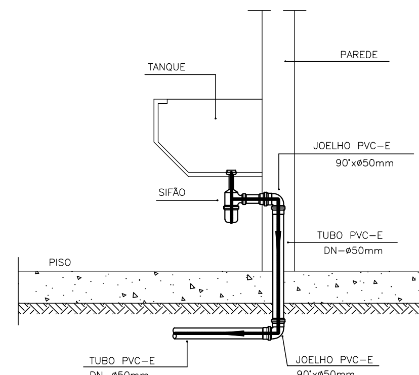
DETALHE DO TANQUE ESCALA 1:25
