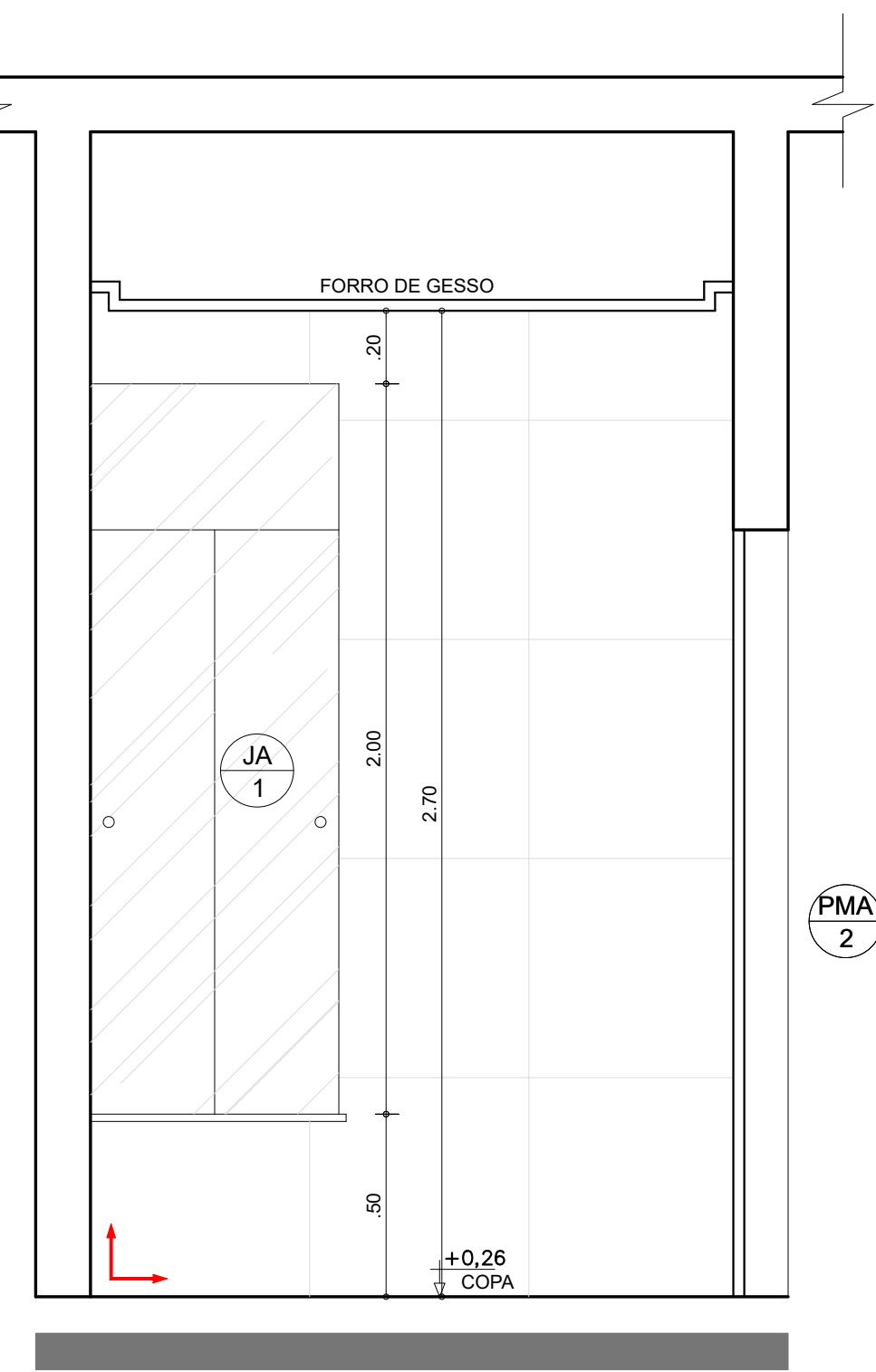
VISTA 4 — COPA PAV. TÉRREO ESC.: 1:25
