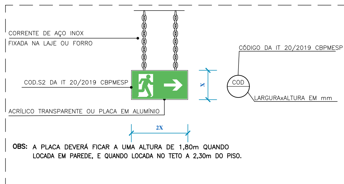
PLACA DE SINALIZAÇÃO DE ABANDONO ESCALA LIVRE
