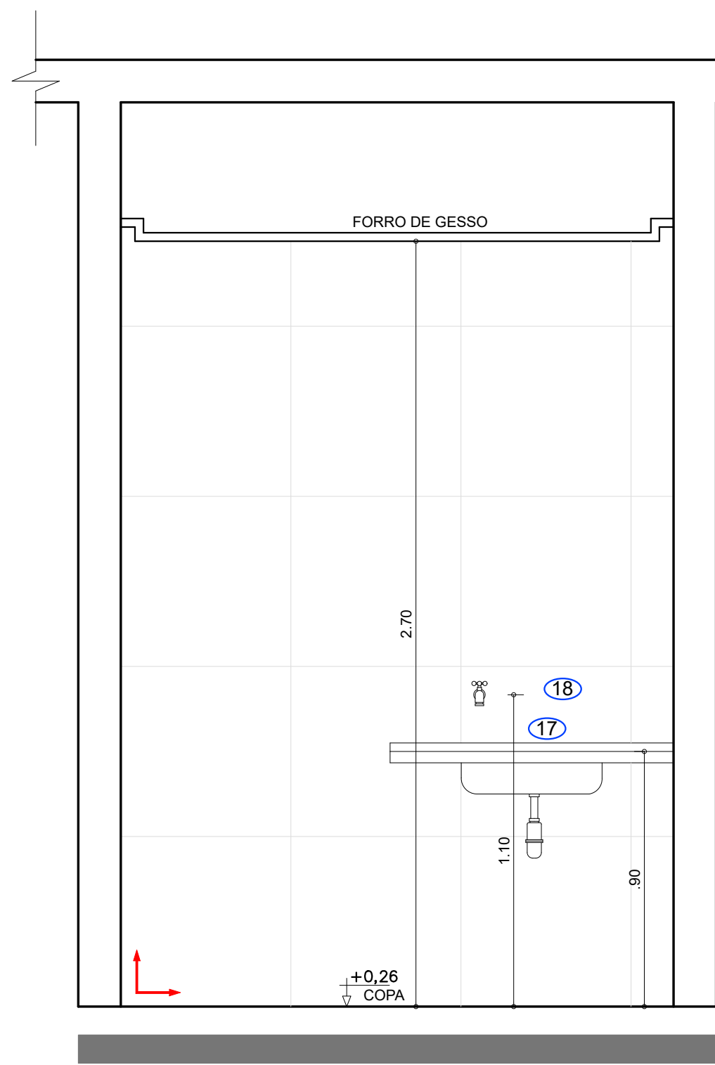
VISTA 3 — COPA PAV. TÉRREO ESC.: 1:25
