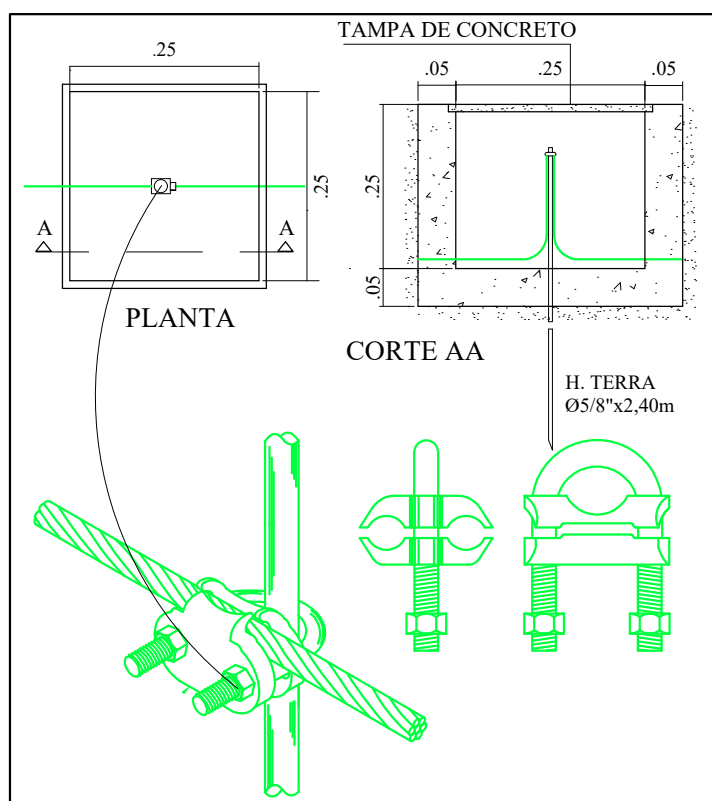
CX. DE INSP. DA H. TERRA S/ ESCALA
