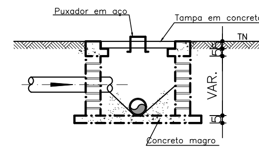
CORTE 1-1
