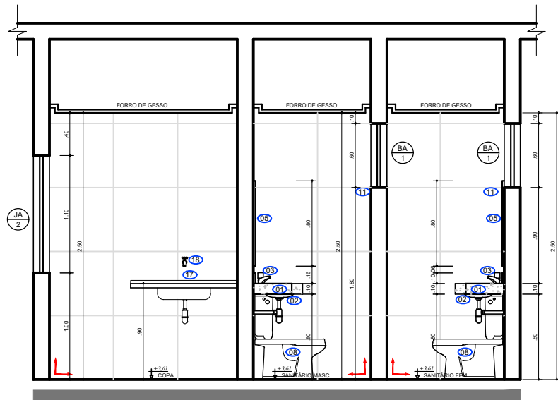
VISTA 2 - SANITÁRIOS PAV. SUPERIOR
