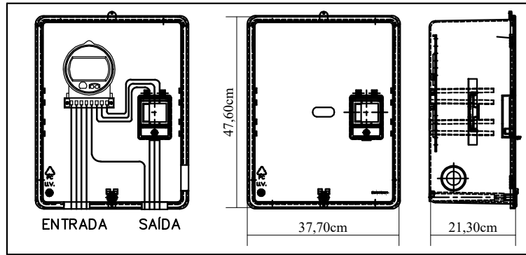
DET. DA CAIXA DE MEDIÇÃO
