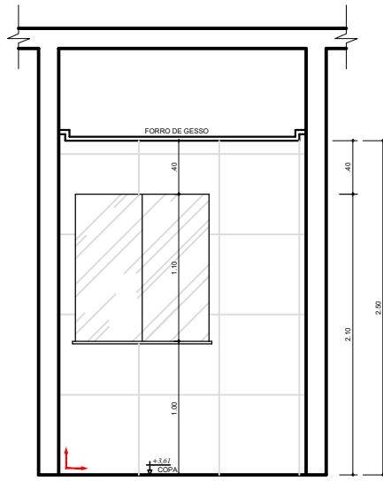
VISTA 7 - SANITÁRIOS PAV. SUPERIOR
