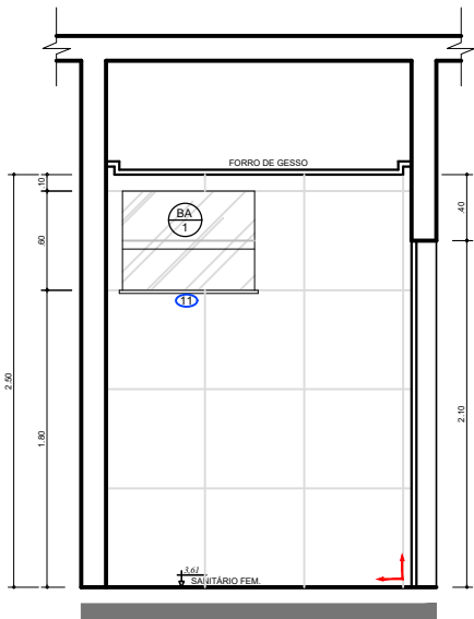
VISTA 3 - SANIT. FEM. PAV. SUPERIOR
