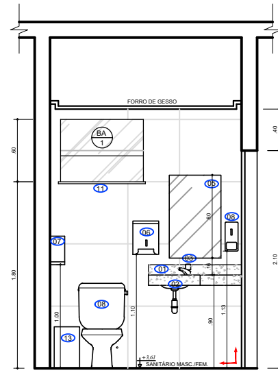
VISTA 4 - SANITÁRIOS PAV. SUPERIOR
